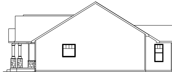
RIGHT ELEVATION
