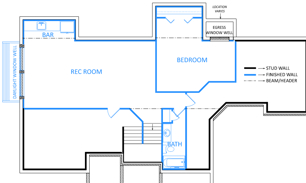
Foundation Option F1 (889 ft 2 )
