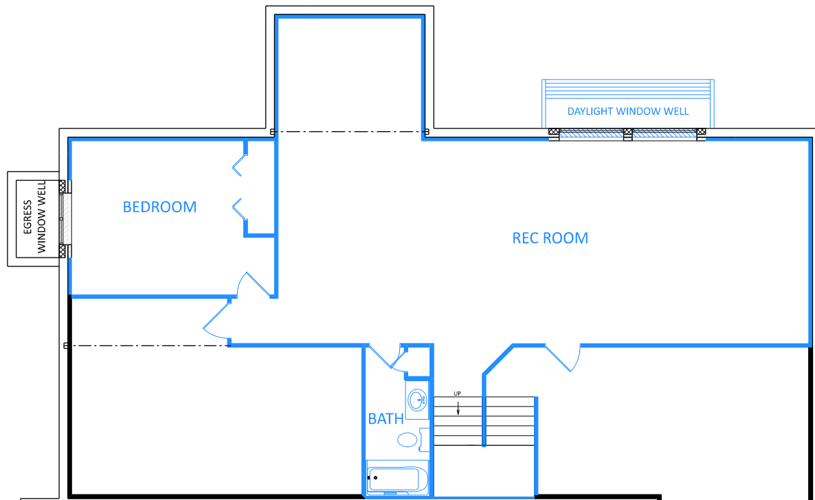
Foundation Option F1 (1,083 ft 2 )
