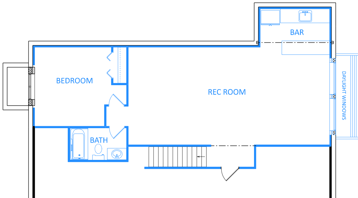
Foundation Option F1 (1,402 ft 2 )
