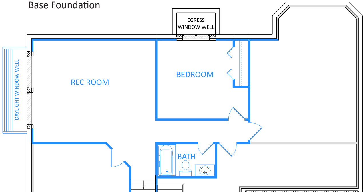
Foundation Option F1 625 sqft
