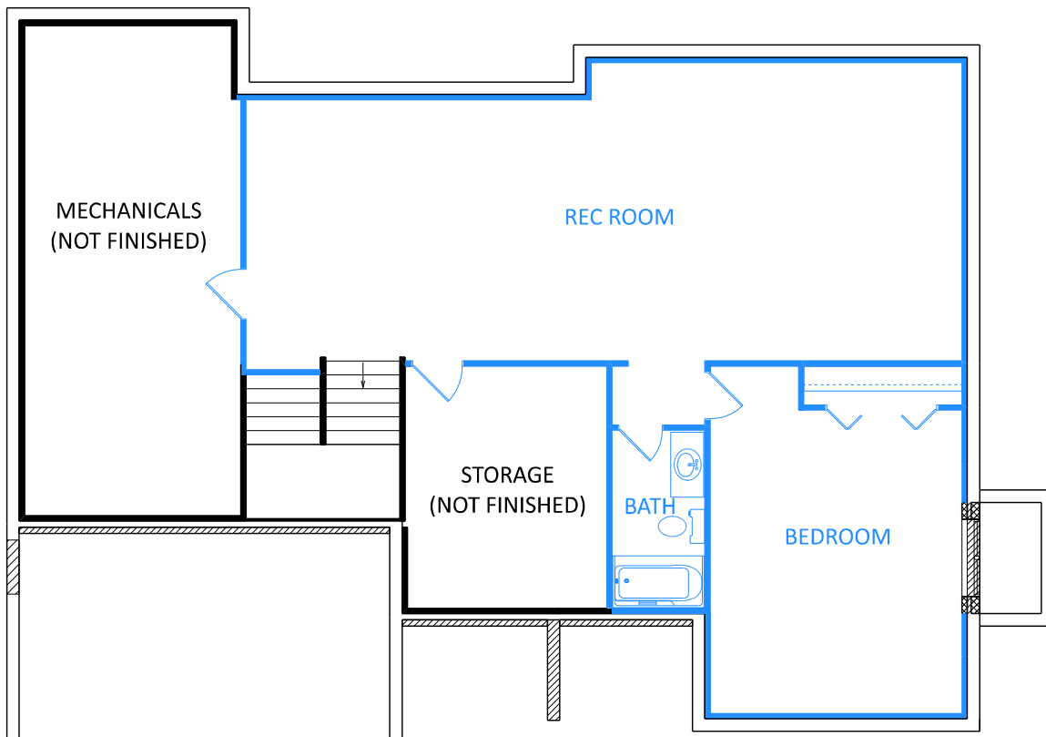
Foundation Option F1 (+954 ft 2 )
