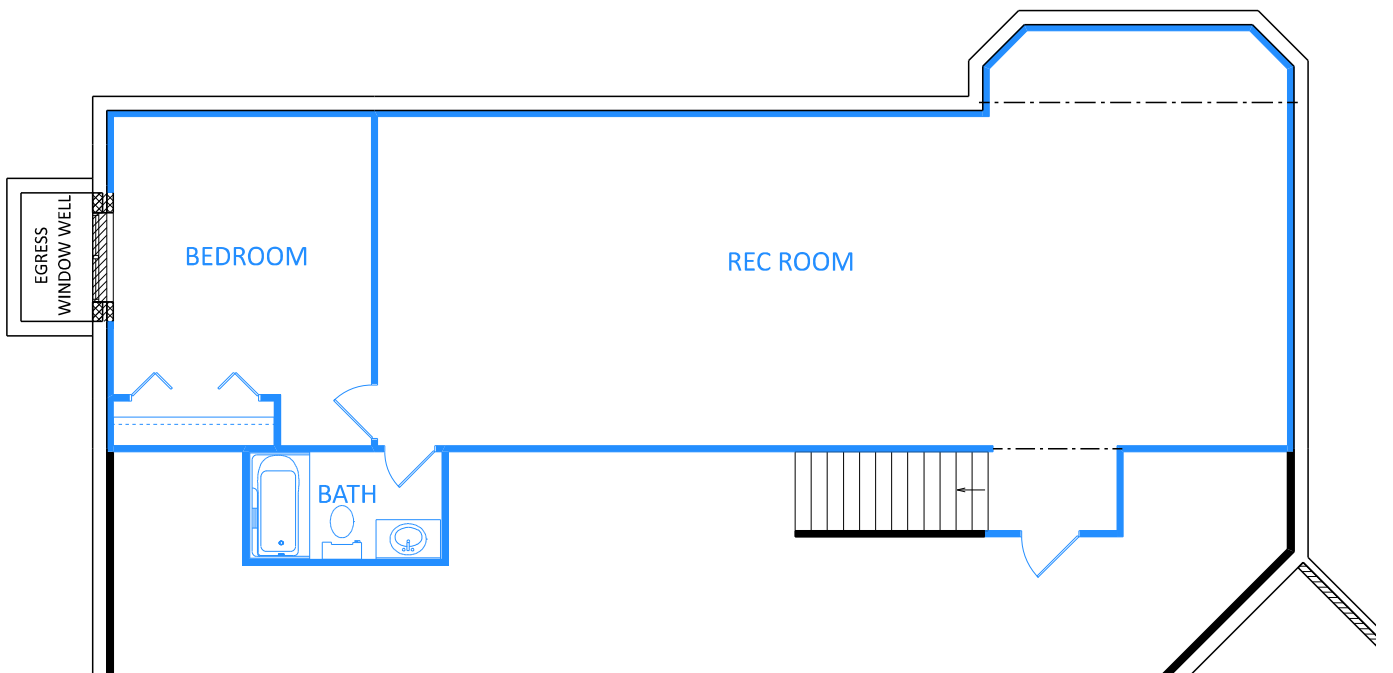
Foundation Option F1 (1,010 ft 2 )
